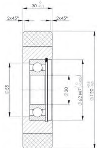
Roller: \phi 120 x 30 art. no. 142 060
